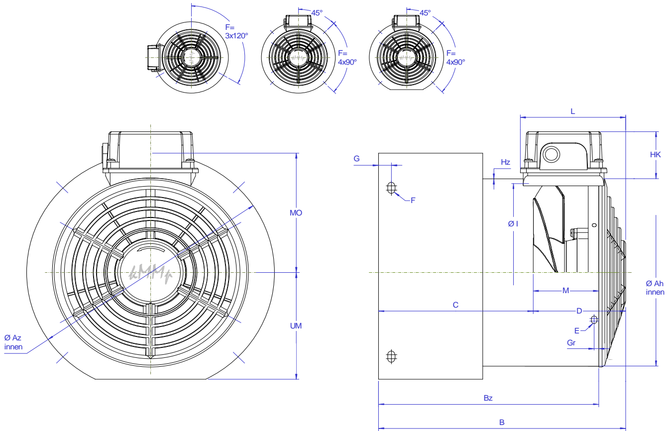
Abmessungen / Dimensions / Côtes / Dimensioni / Cotas
